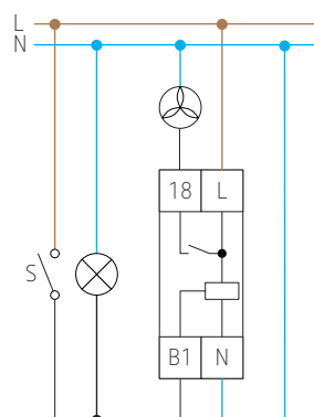
Commande d'une lampe et d'un ventilateur
