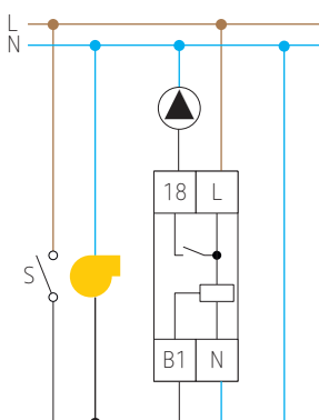
Commande d'un brûleur et d'un circulateur
