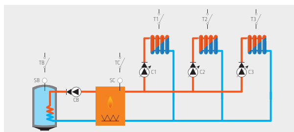
SWW-productie zonder kraan
