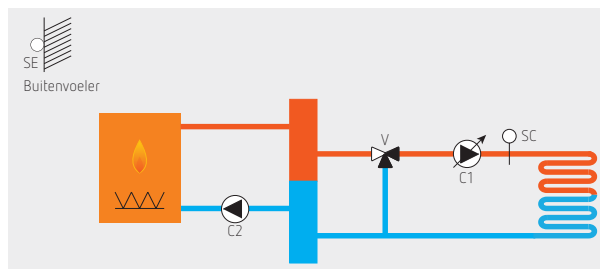
Weersafhankelijke regeling zonder sturing van SWW-productie
